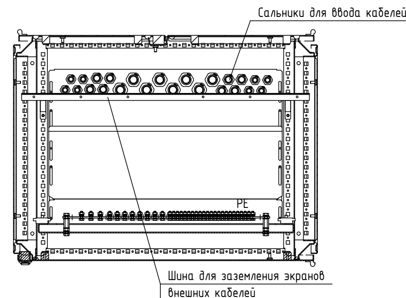
Б-Б
