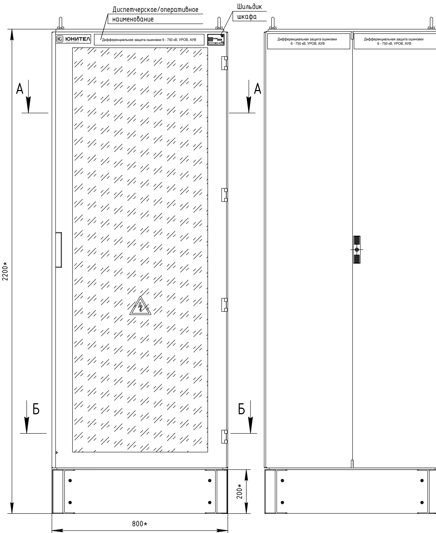
Вид сзади
